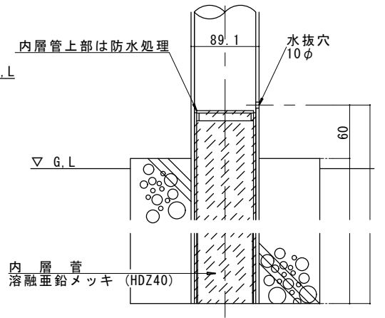
塩害対策主柱脚断面図 (1/5)
