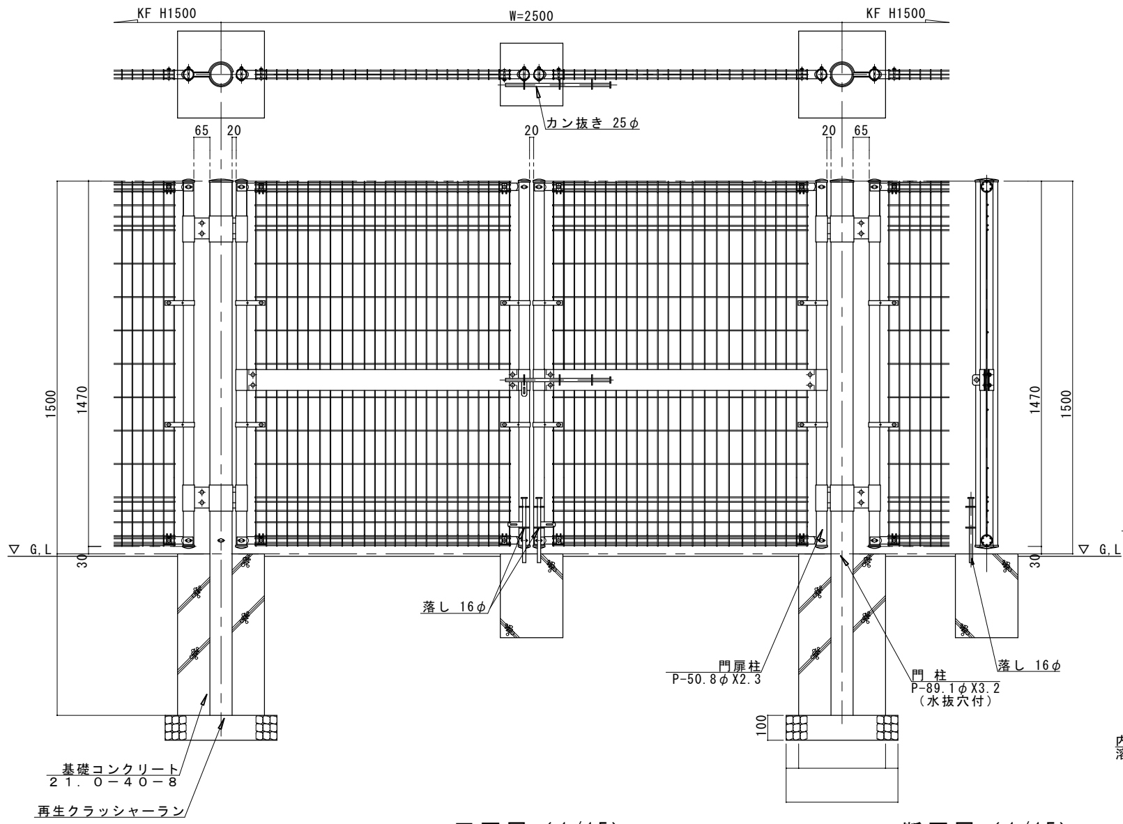
正面図 (1/15)
